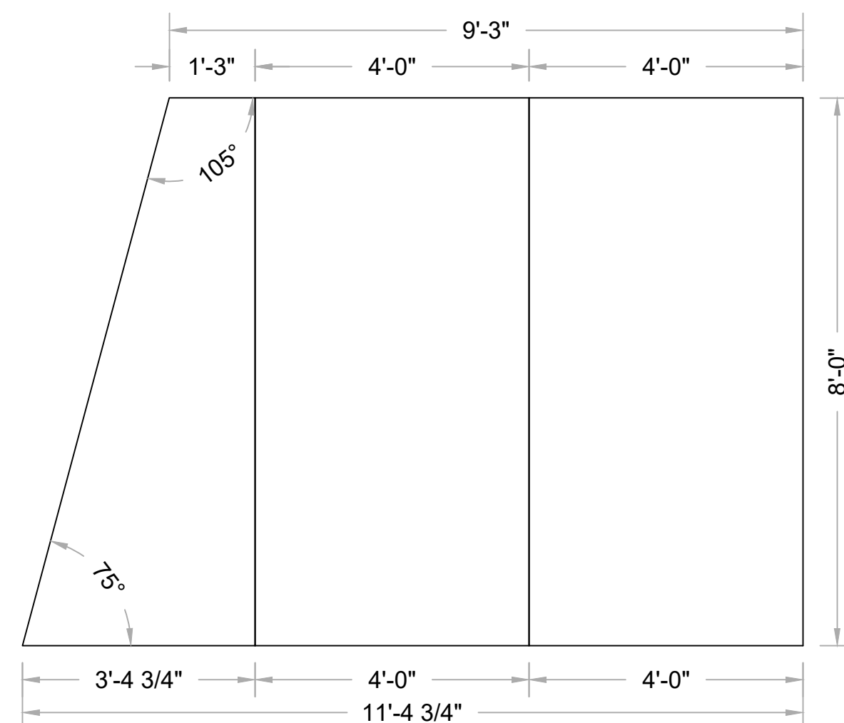
2 FRONT Scale: 1/2" = 1'-0"
