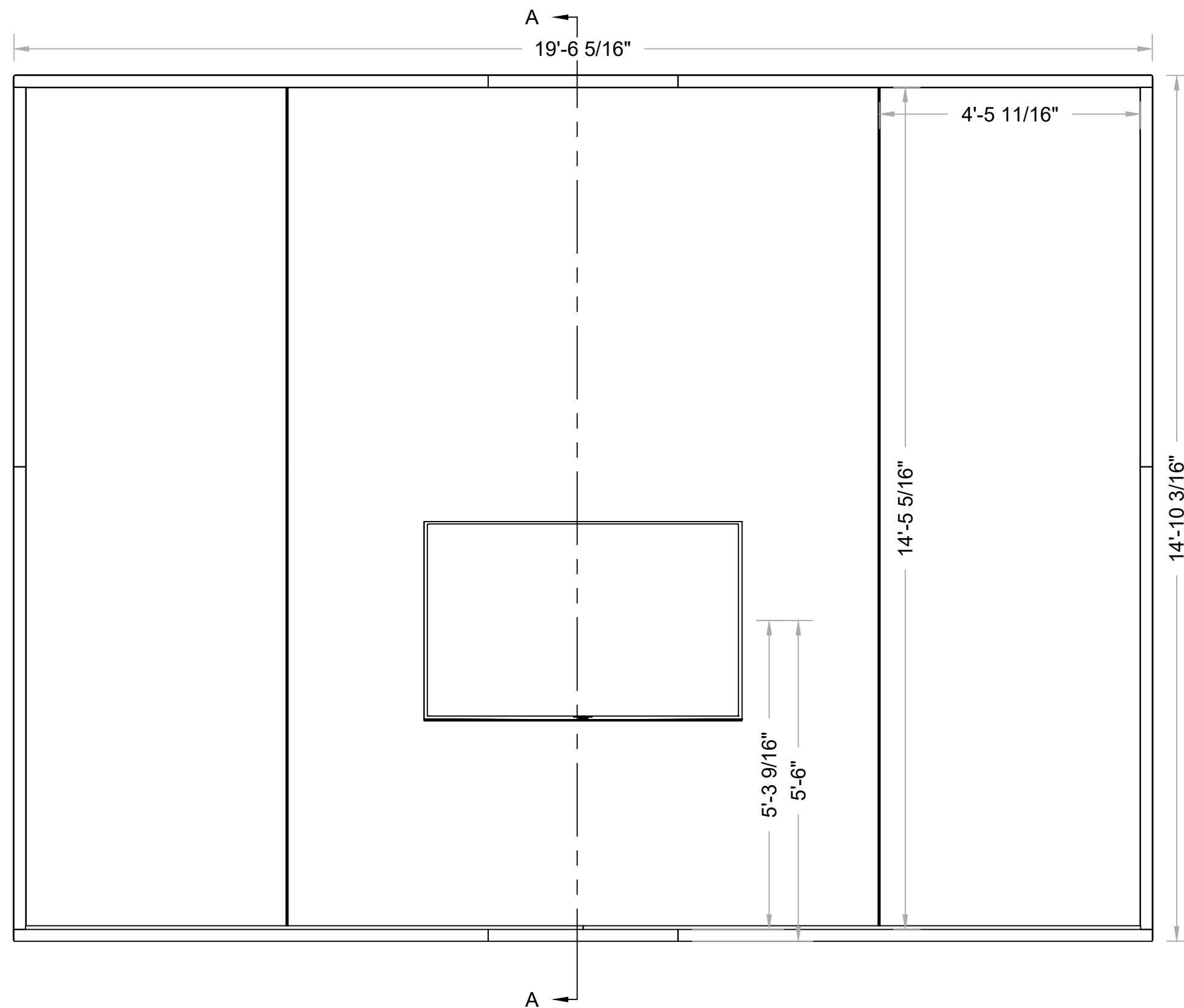
2 FRONT Scale: 1/2" = 1'-0"
