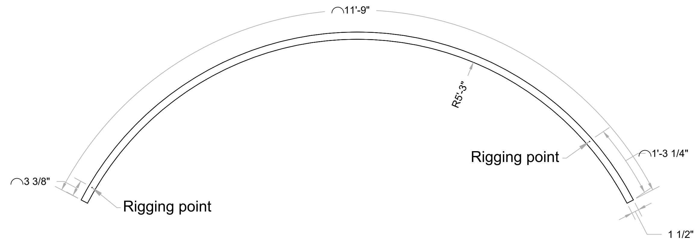
1 TOP Scale: 1" = 1'-0"
