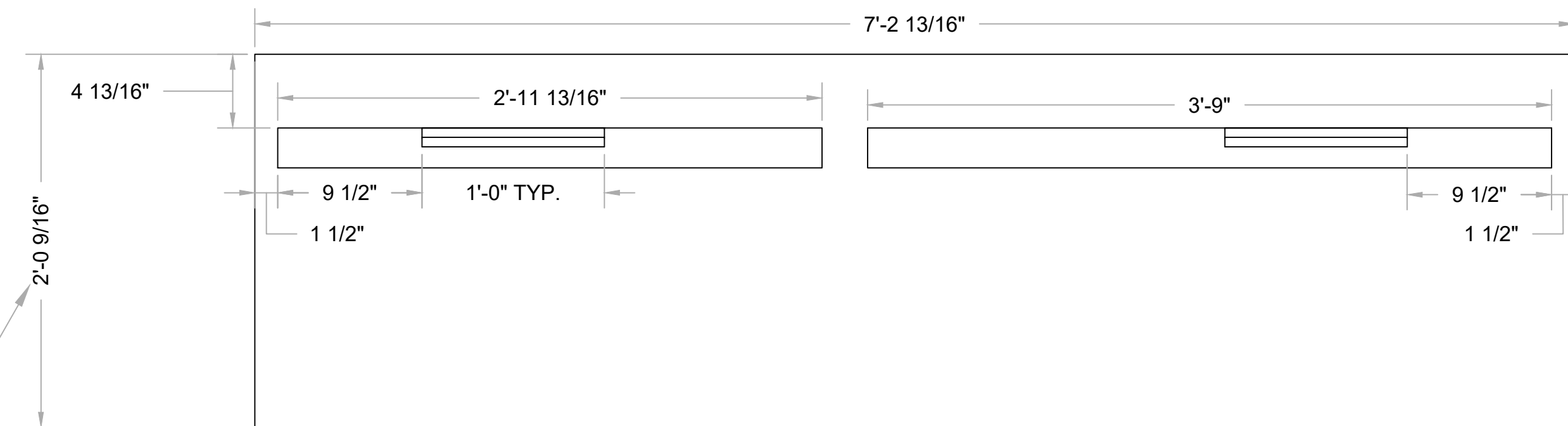
4 BACK Scale: 1-1/2" = 1'-0"
