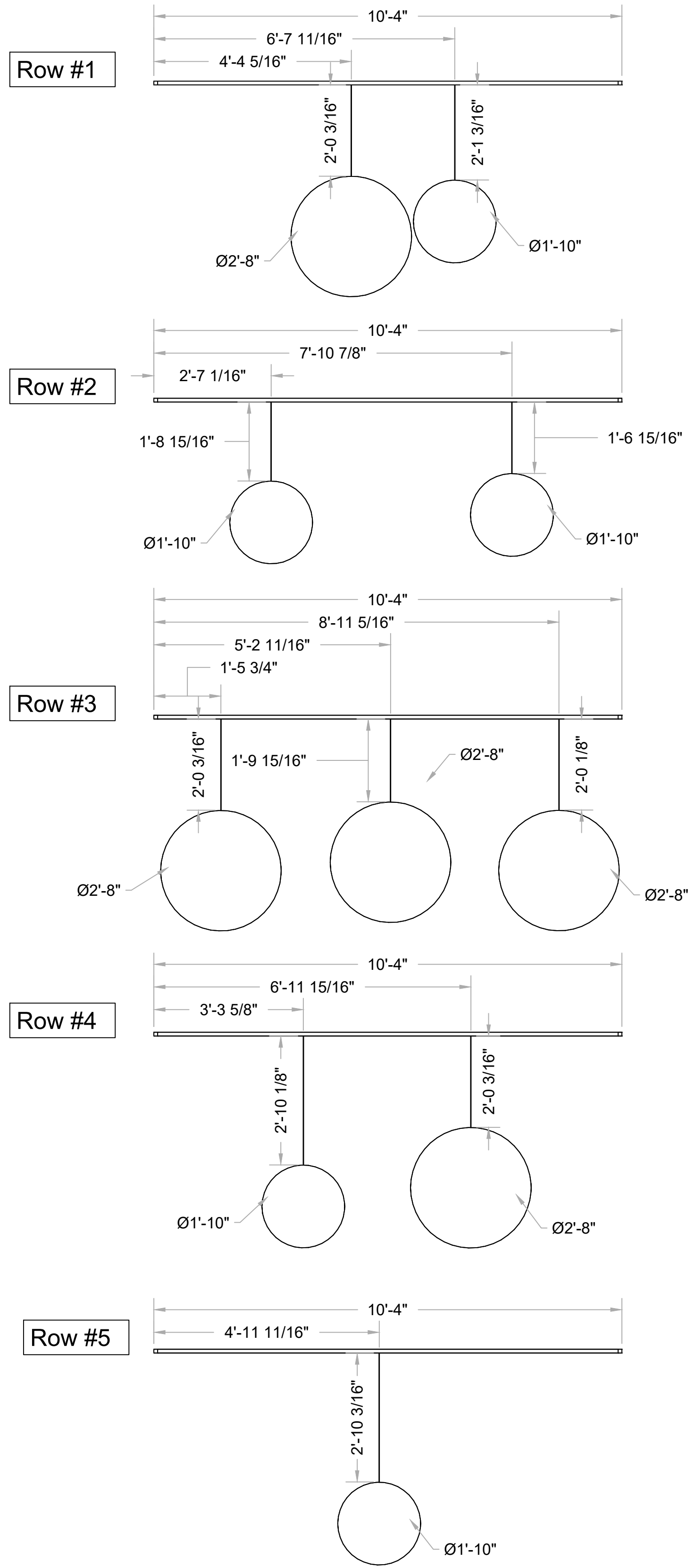
1 FRONT Scale: 1/2" = 1'-0"
