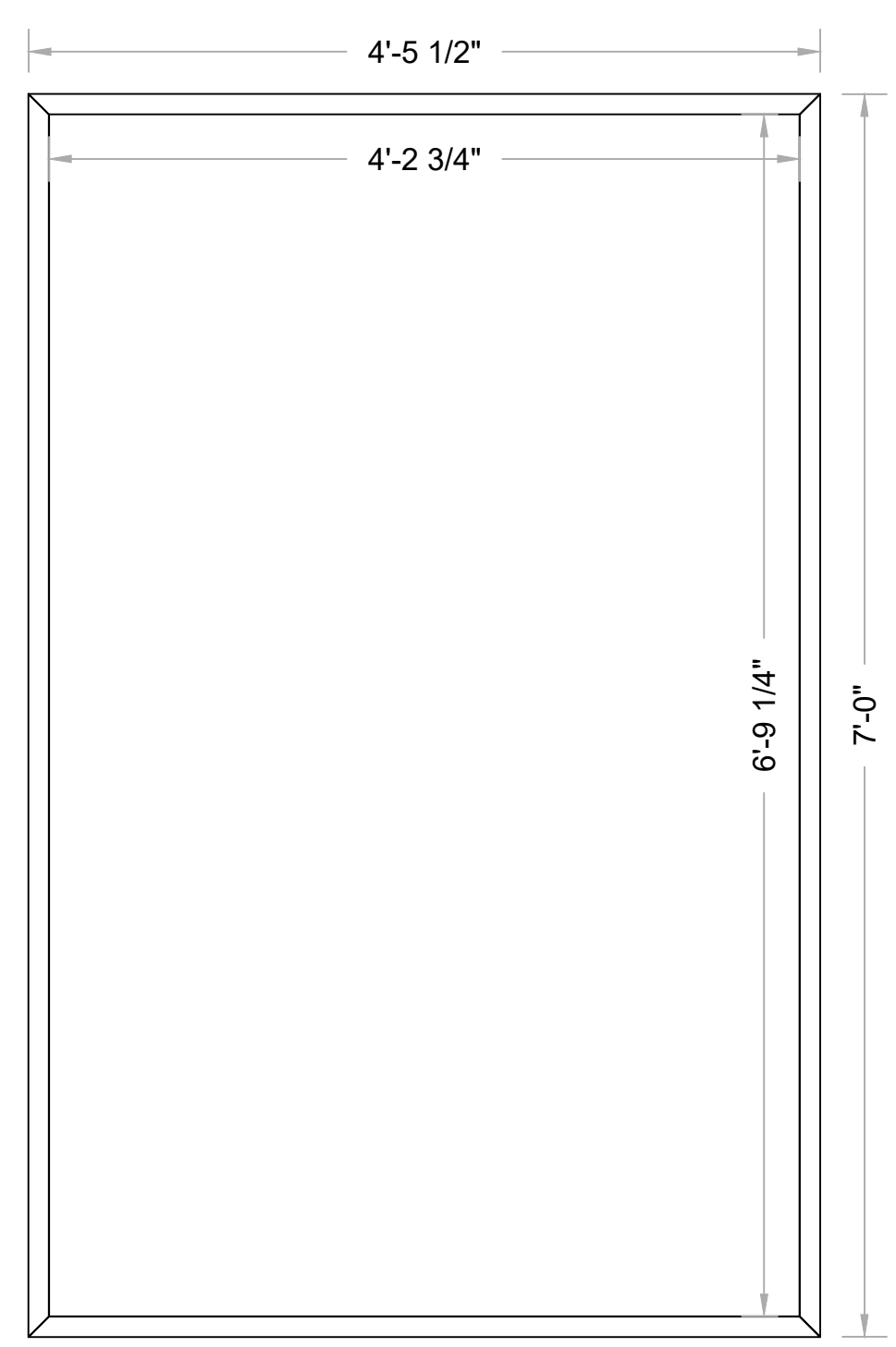
2 FRONT Scale: 1" = 1'-0"
