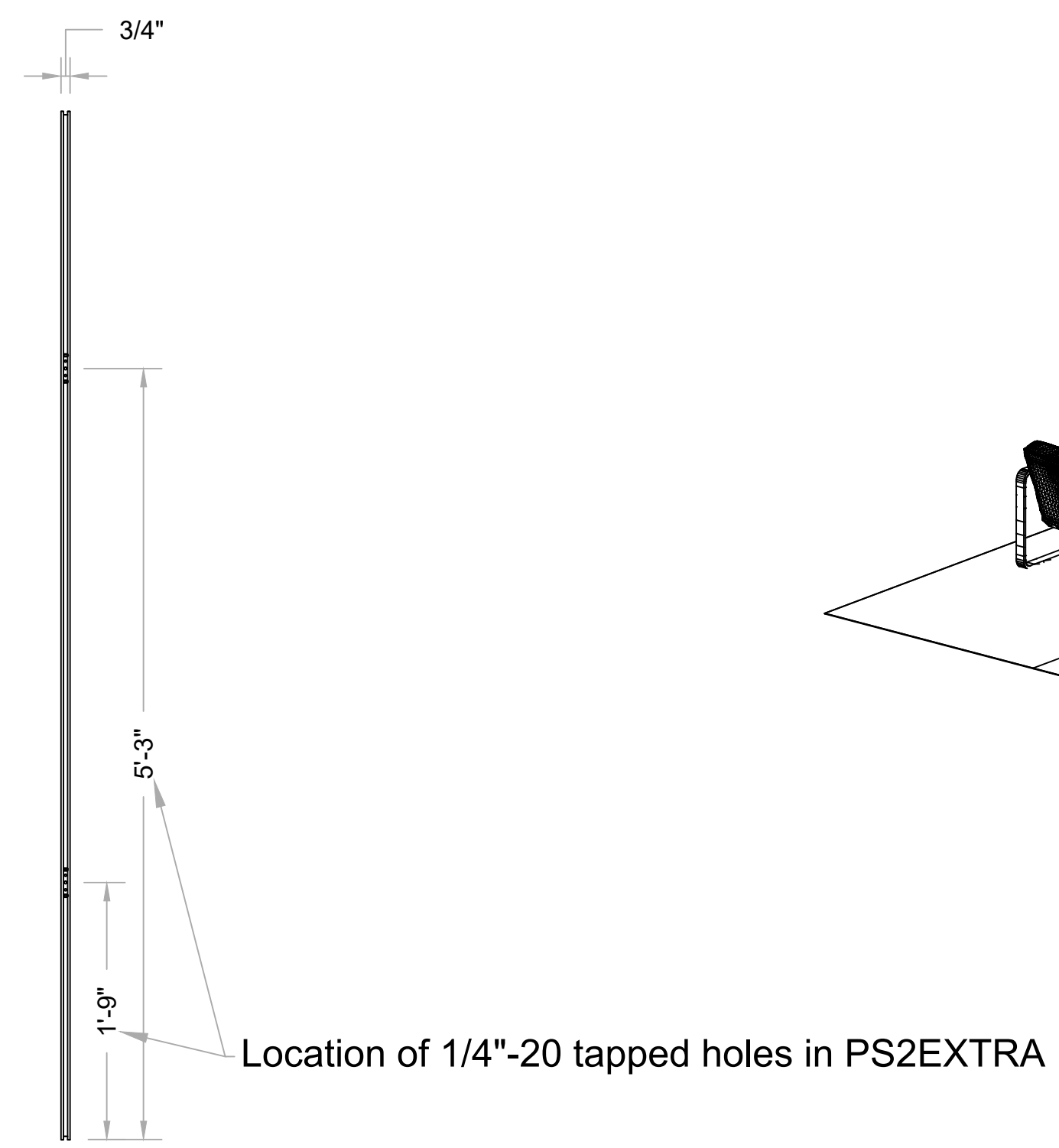
3 RIGHT Scale: 1" = 1'-0"
