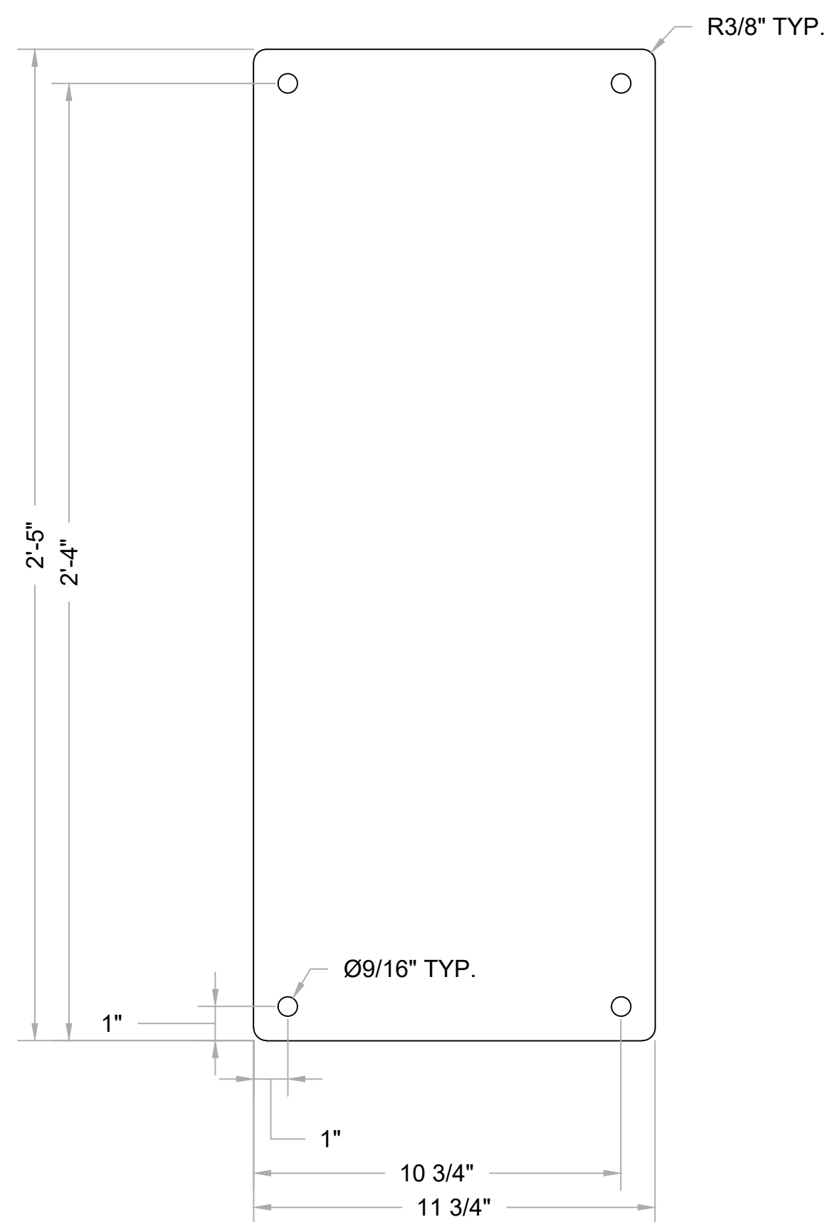
2 FRONT Scale: 3" = 1'-0"
