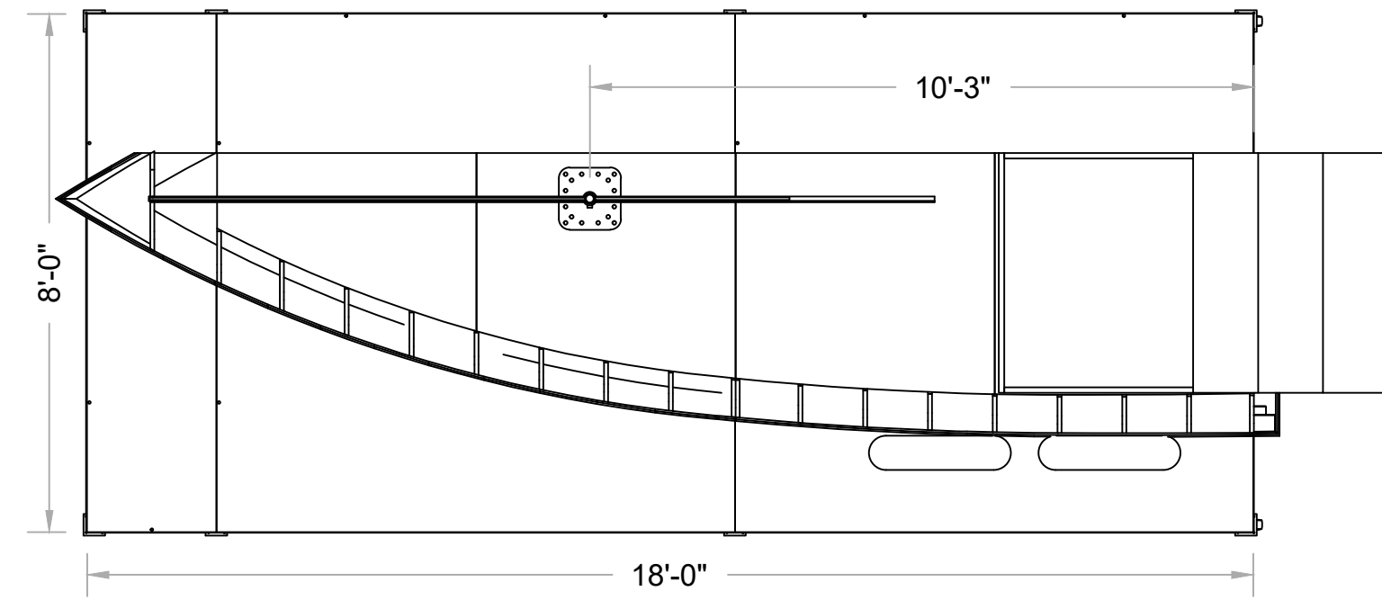
1 TOP Scale: 3/8" = 1'-0"
