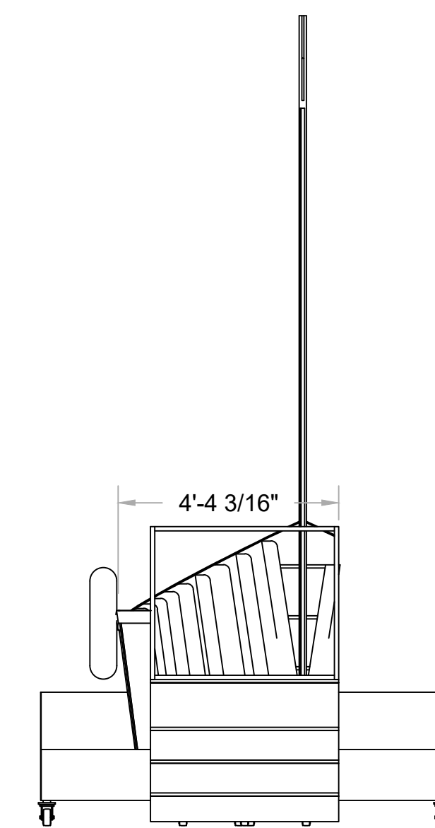
3 RIGHT Scale: 3/8" = 1'-0"
