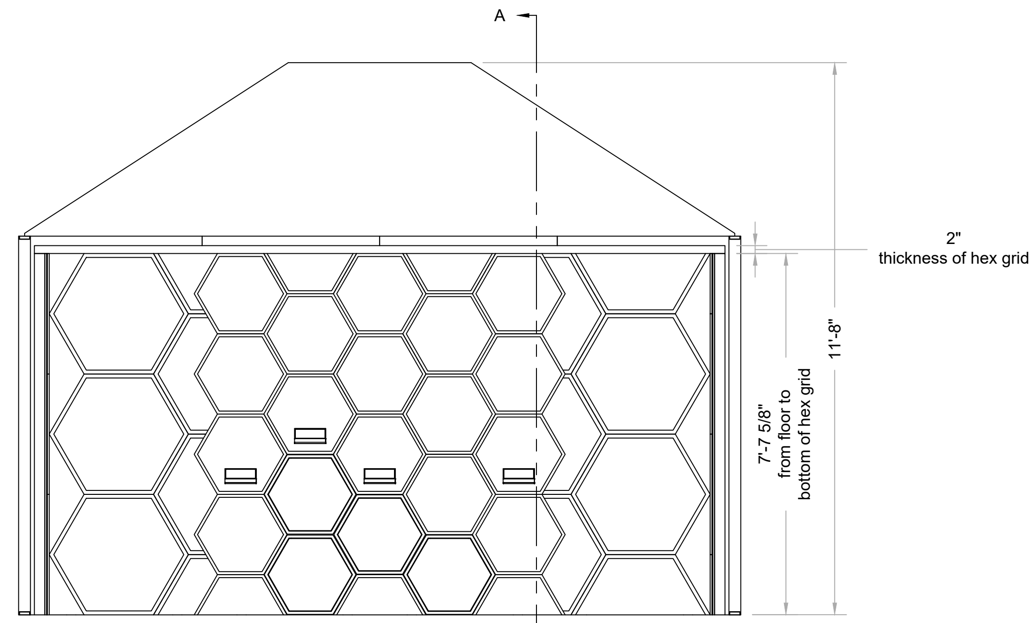
2 FRONT Scale: 1/2" = 1'-0"
