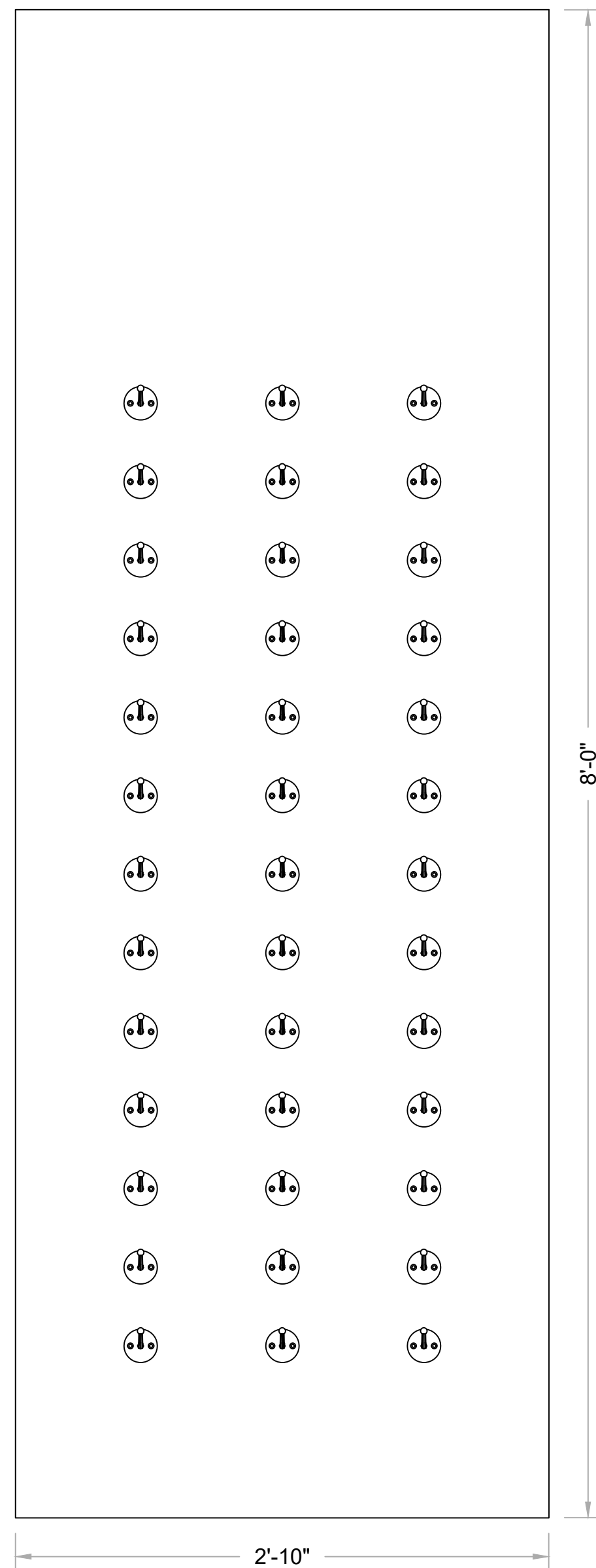
2 FRONT Scale: 1-1/2" = 1'-0"
