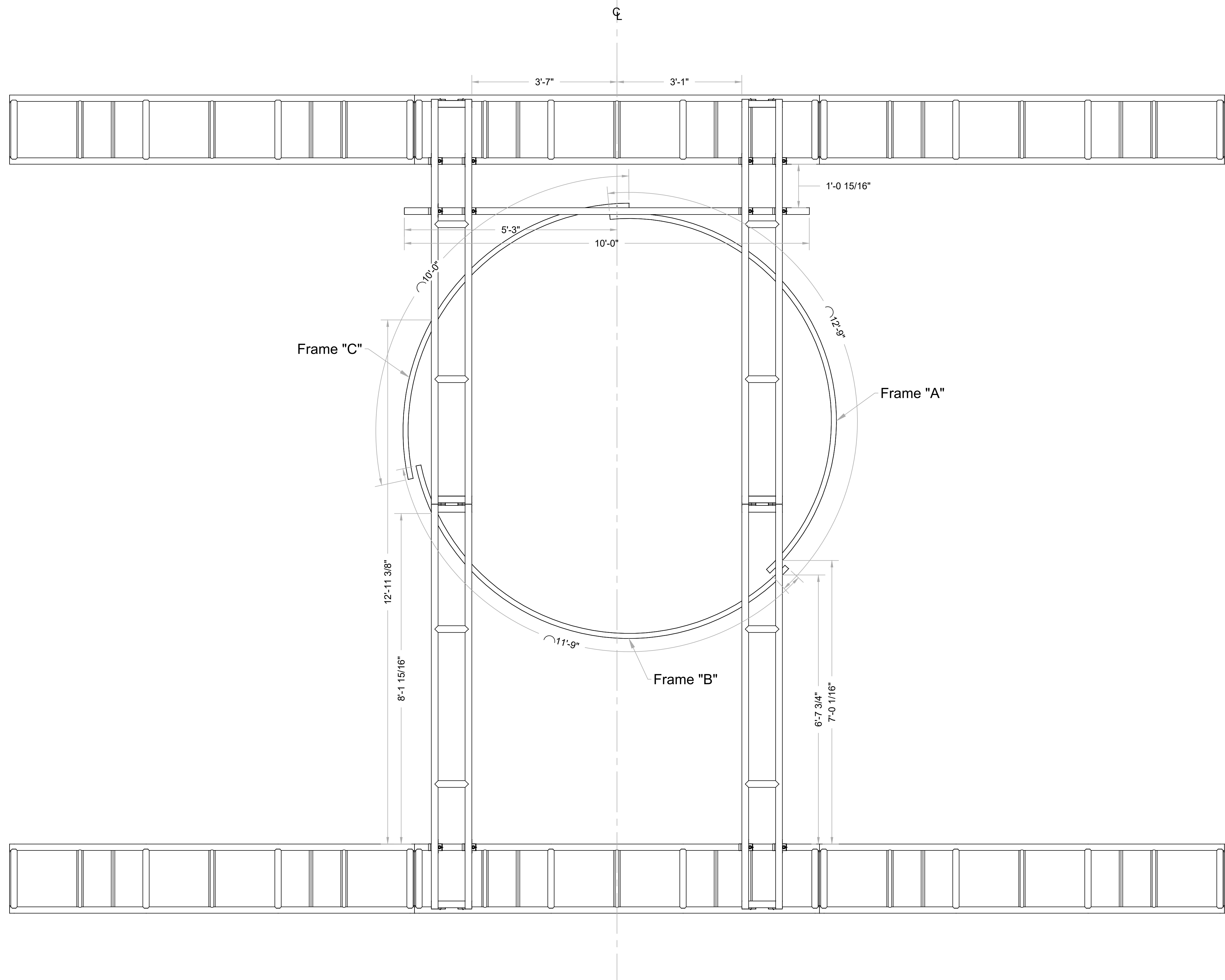
1 TOP Scale: 3/4" = 1'-0"
