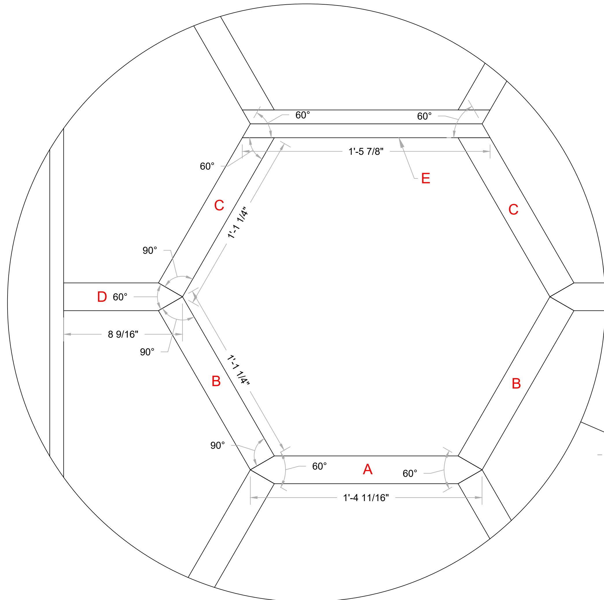
DETAIL G Scale: 3" = 1'-0"
