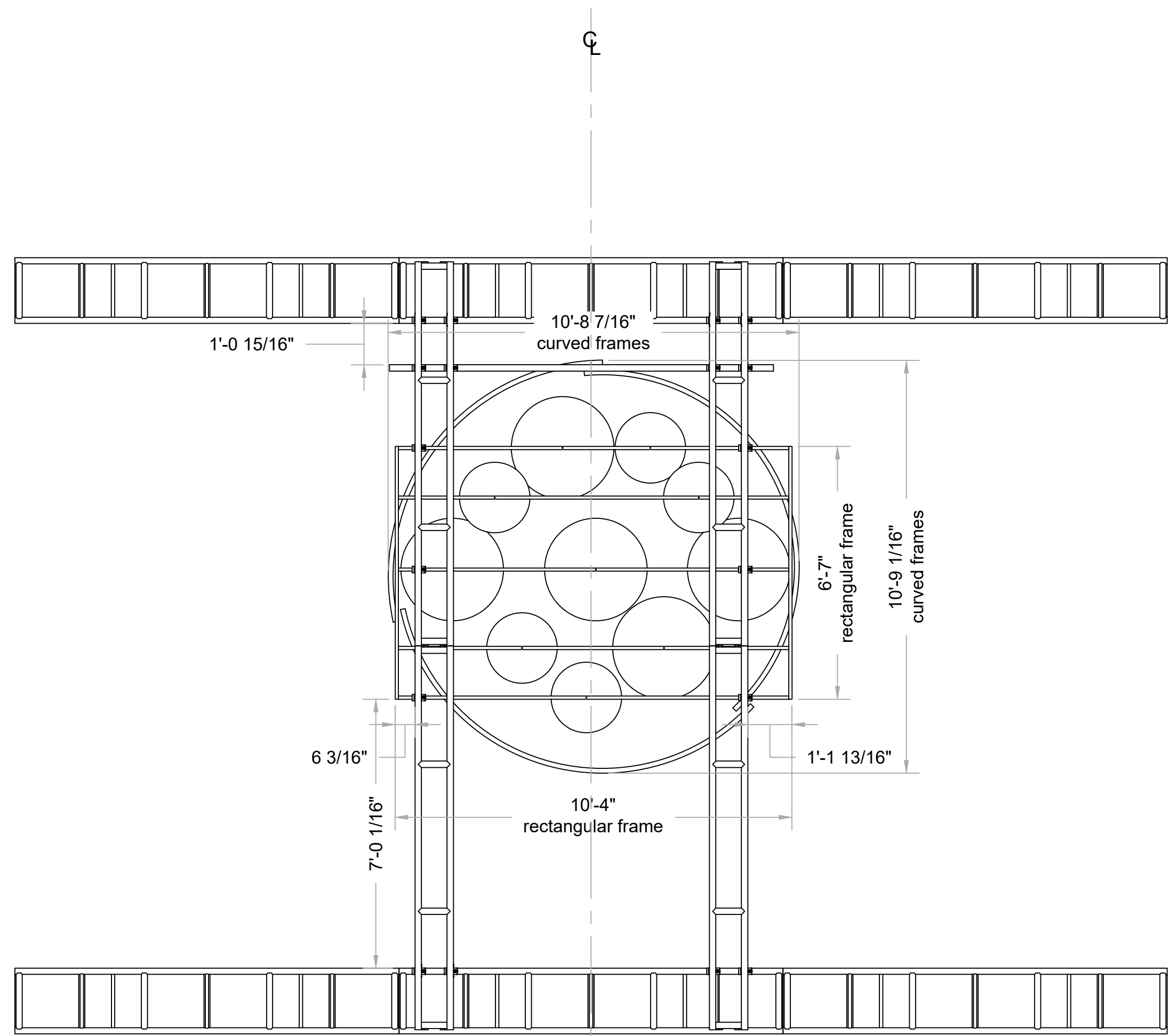
1 TOP Scale: 3/8" = 1'-0"
