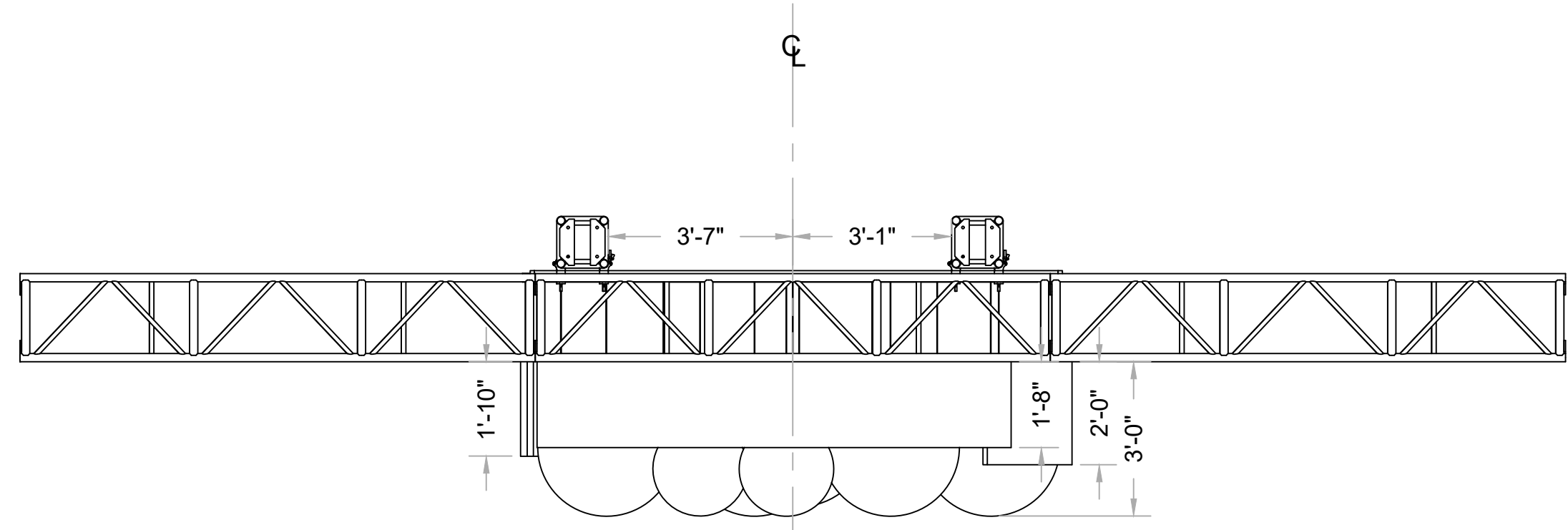
2 FRONT Scale: 3/8" = 1'-0"
