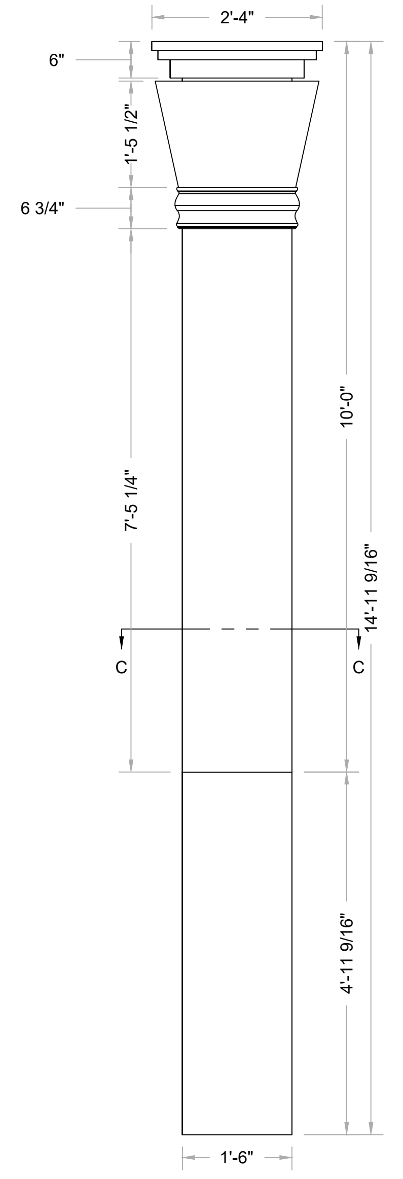
3 FRONT Scale: 3/4" = 1'-0"
