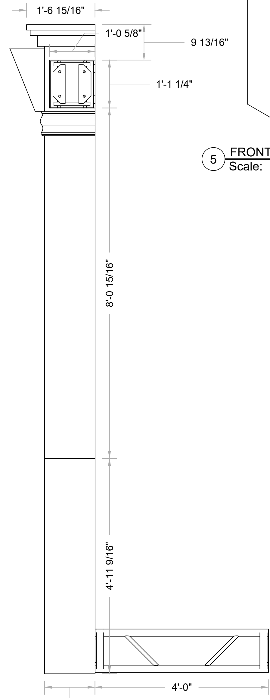
4 RIGHT Scale: 3/4" = 1'-0"
