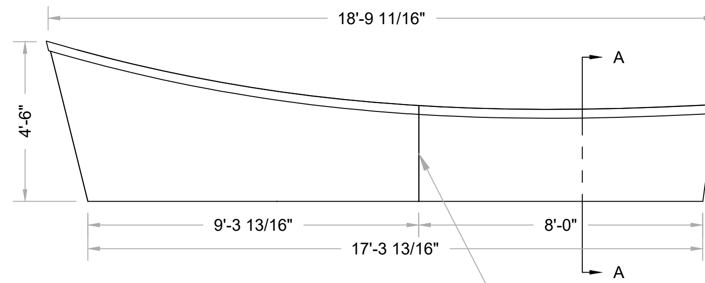
2 FRONT Scale: 3/8" = 1'-0"
