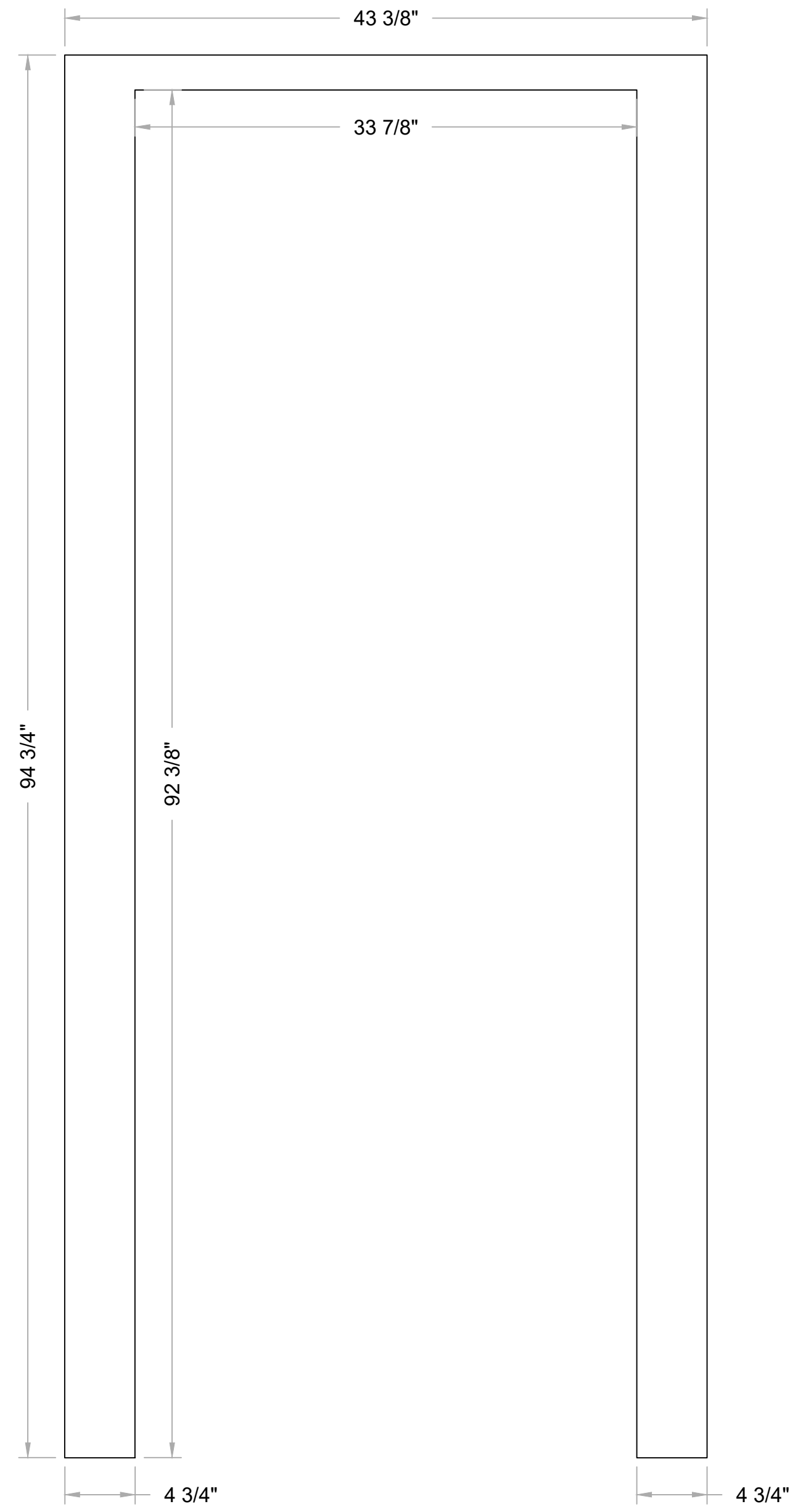
2 SEG3a FRONT VIEW Scale: 1-1/2" = 1'-0"
