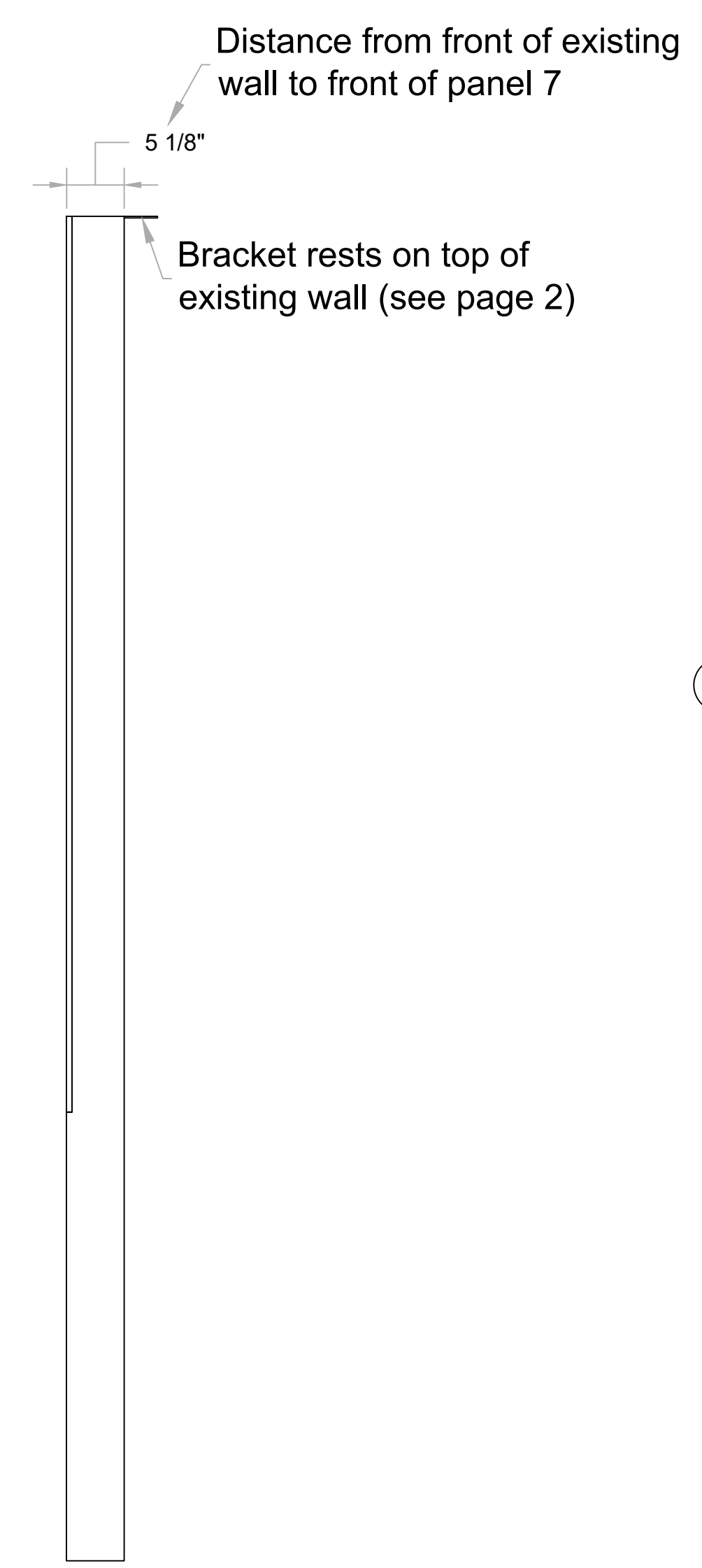
4 RIGHT Scale: 1" = 1'-0"
