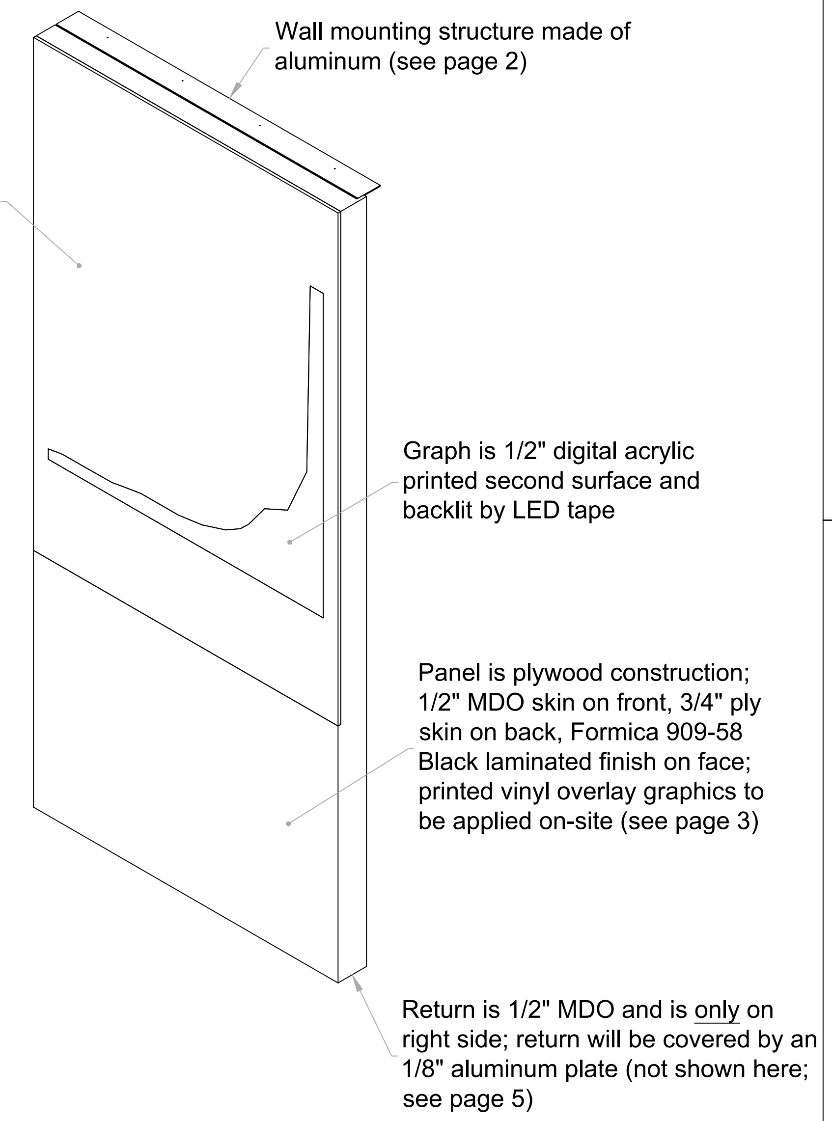
5 FRONT ISO Scale: NTS
