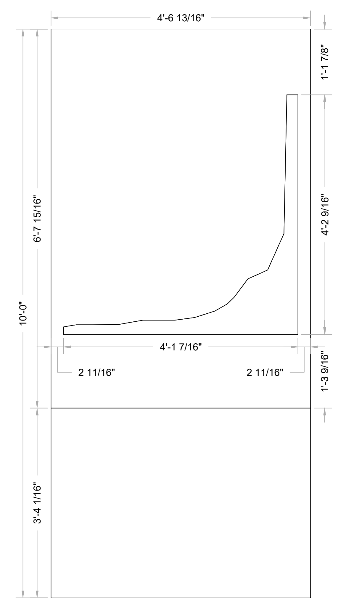
3 FRONT Scale: 1" = 1'-0"
