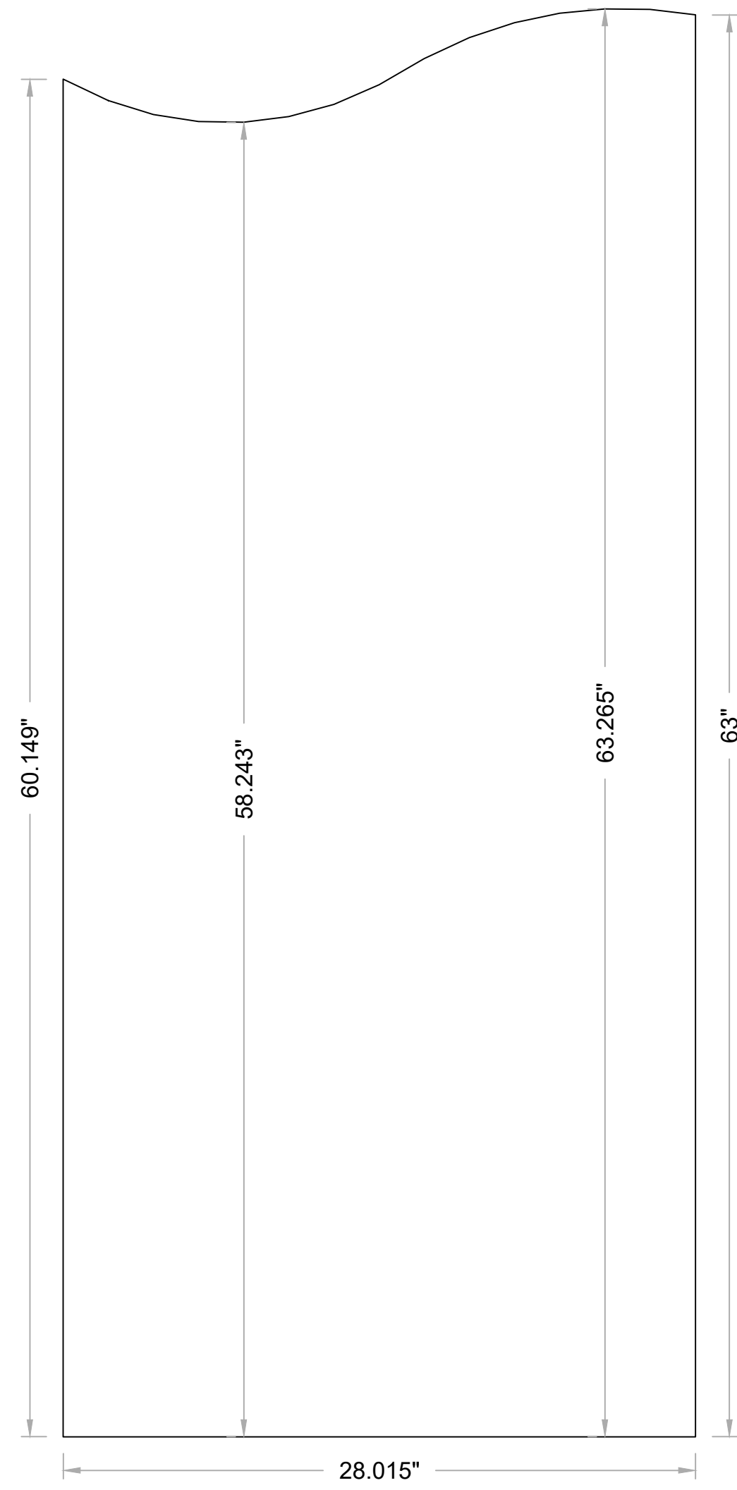
1 FRONT SKIN Scale: 1-1/2" = 1'-0"
