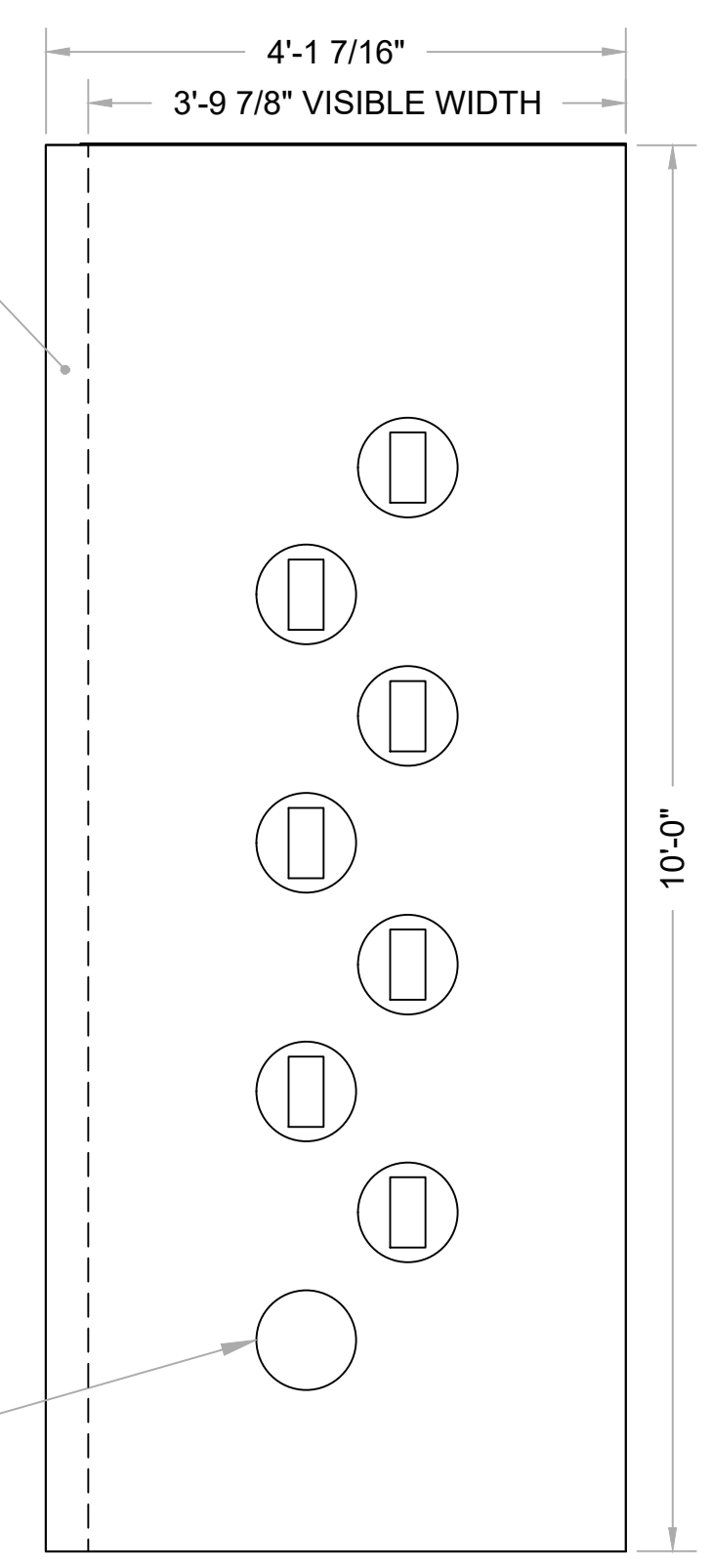
2 FRONT Scale: 3/4" = 1'-0"
