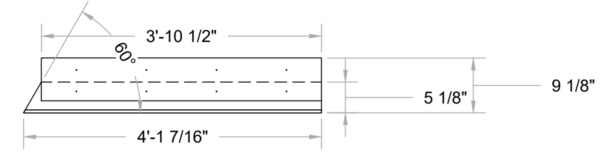
1 TOP Scale: 3/4" = 1'-0"
