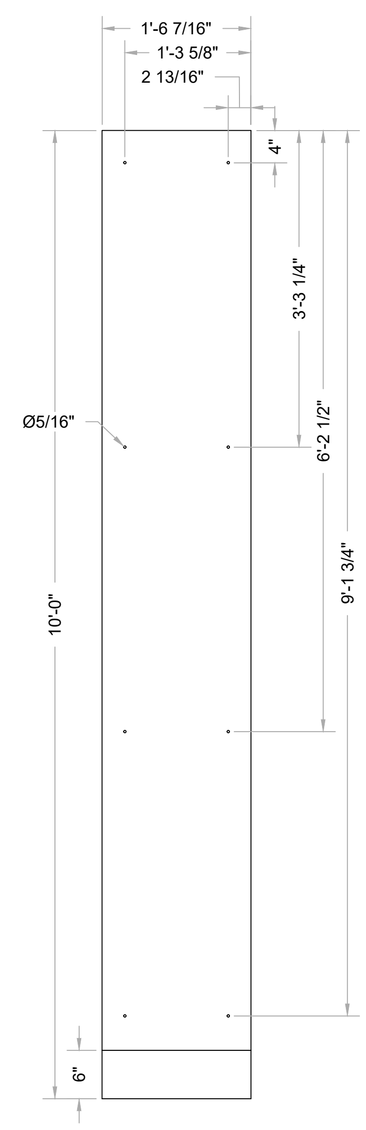
2 TOP Scale: 1" = 1'-0"
